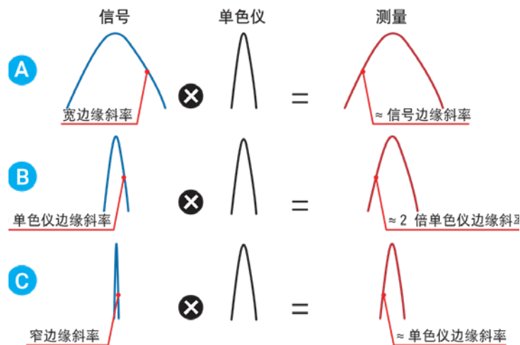
图6：信号和单色仪形状卷积示意图。
