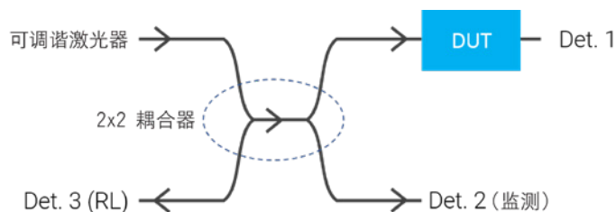
图8：典型的IL和RL测量设置。
