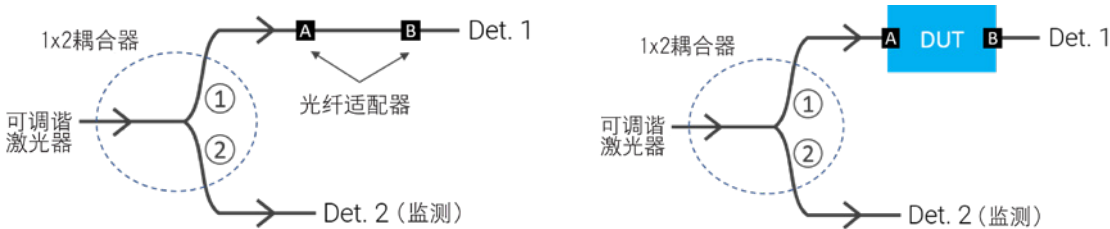
图2：两步测试流程。 步骤1（左）：不使用DUT进行基准测量。步骤2（右）：使用DUT进行测量。
