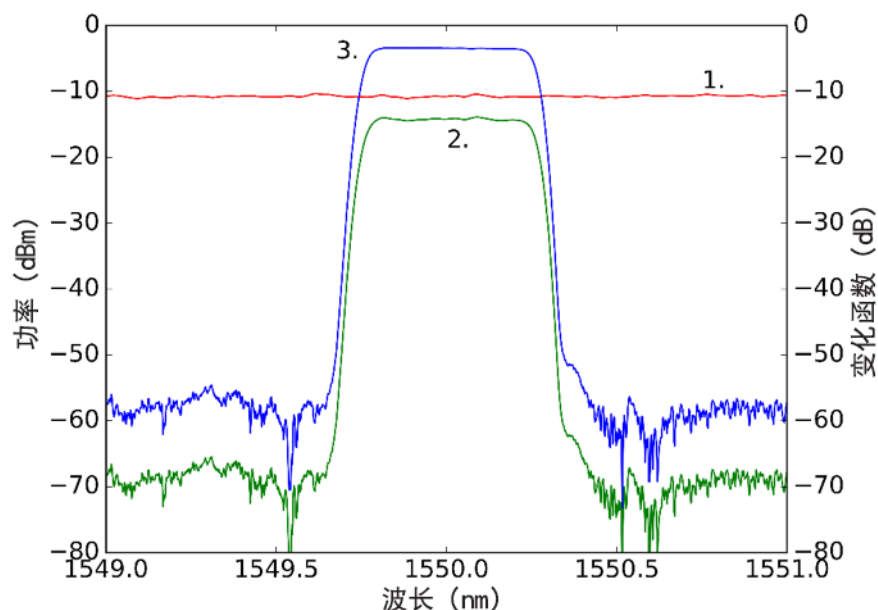
图5：使用宽带光源和OSA鉴定滤波器。
